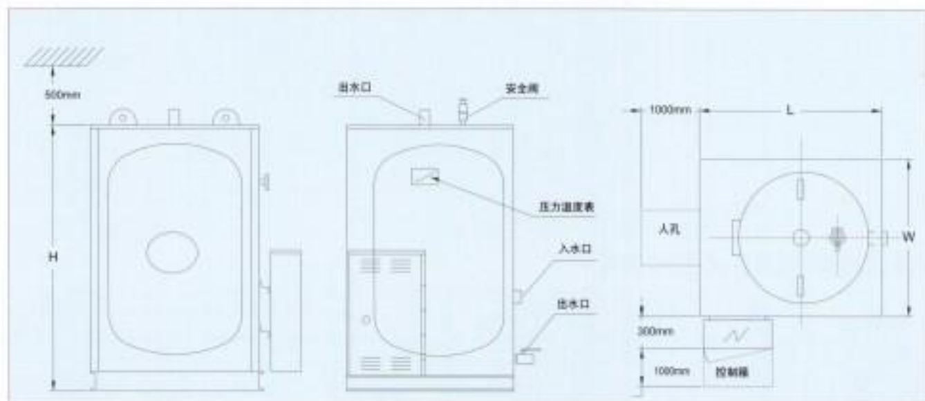
新波能牌 EHWC系列(储水式立式)电热水炉示意图
